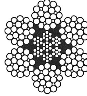
6 x 25 Filler IWRC
